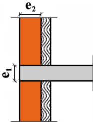
شکل پ ۱۰-۱۱ اتصالات متداول سقف‌های میانی
